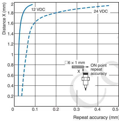
E2E-C03N02□/E2E-S04N02□
