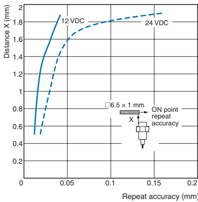
E2E-C06S02□
