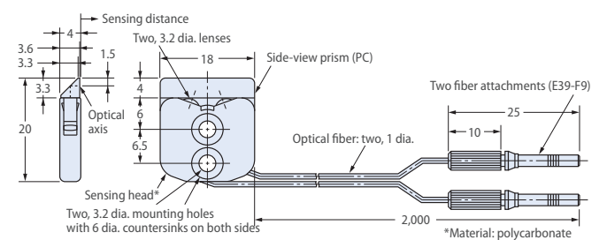
E32-L25
