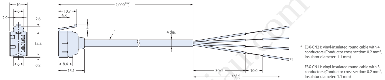
E3X-CN22/E3X-CN12 (slave connector)
