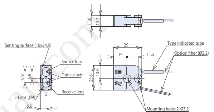
E32-L16-N
