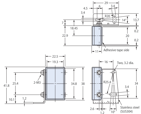
E39-R3
