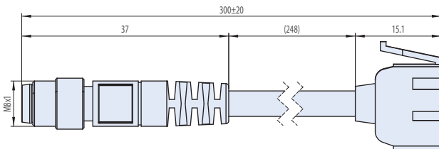
E3X-CN21-M3J-02 0.3M
