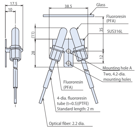
E32-L11FS
